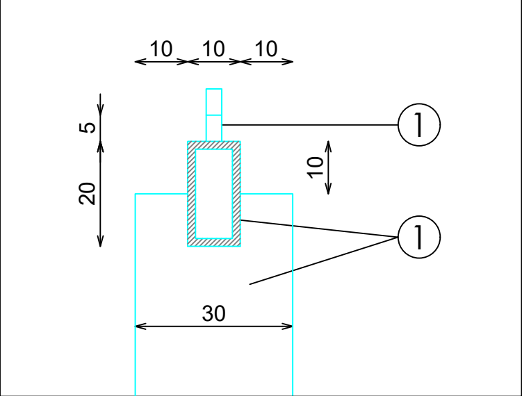
DETALLE B
