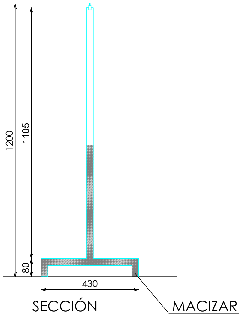
SECCIÓN
