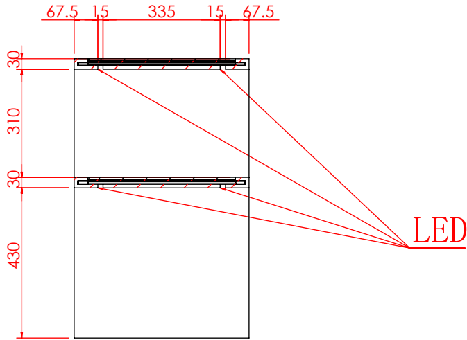
剖面 AG-AG
