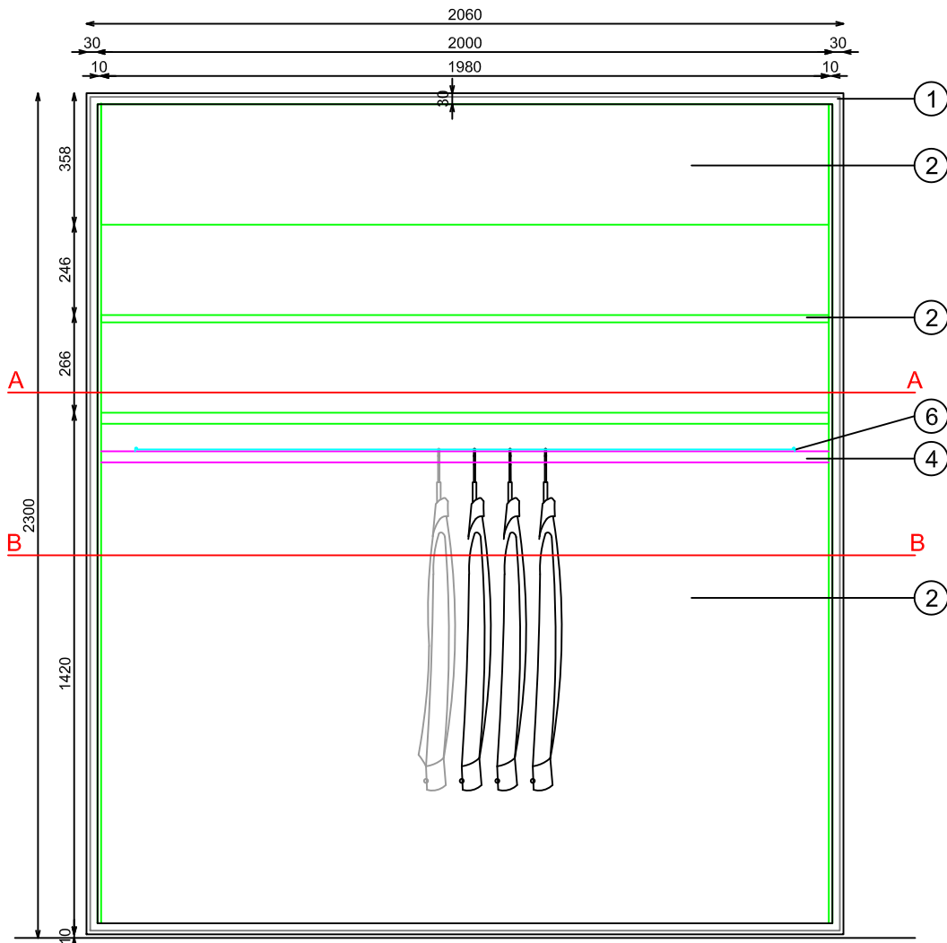
ALZADO FRONTAL
