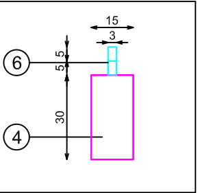
DETALLE BARRA
