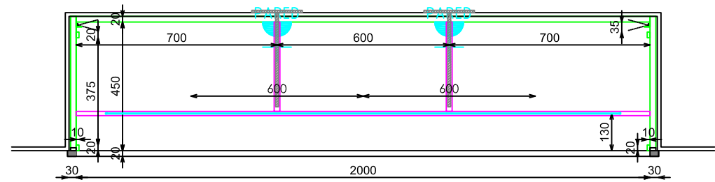
PLANTA B-B
