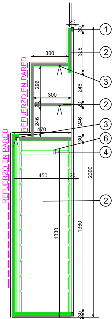
SECCION
