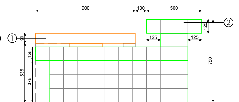
ALZADO LATERAL
