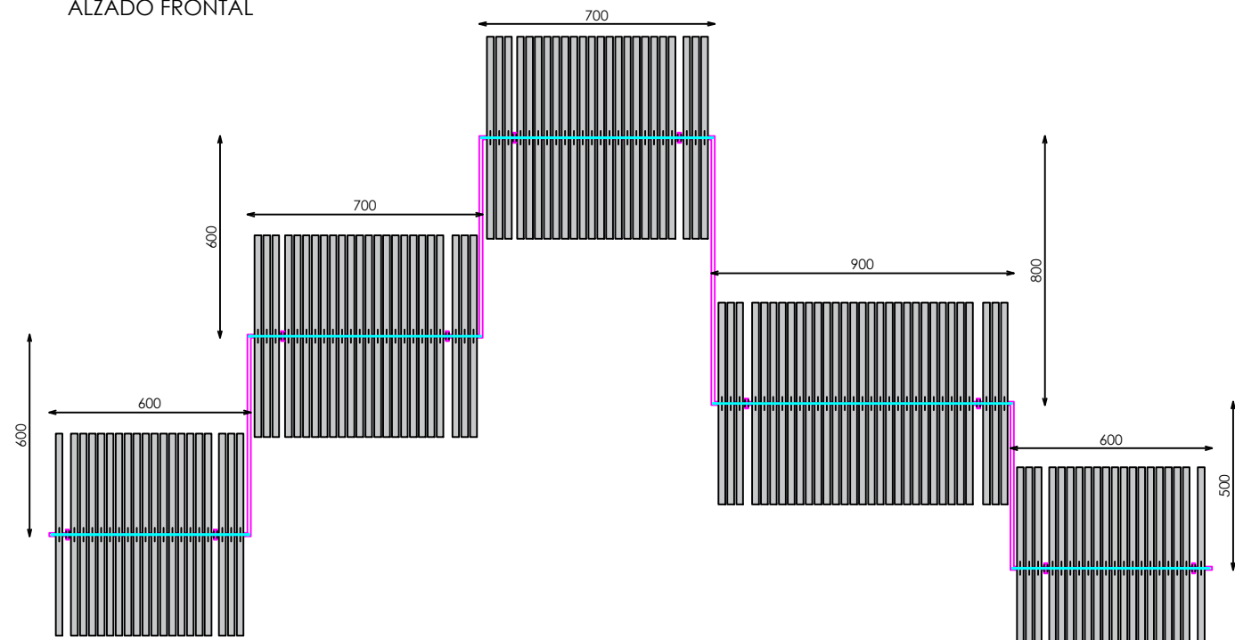
PLANTA
