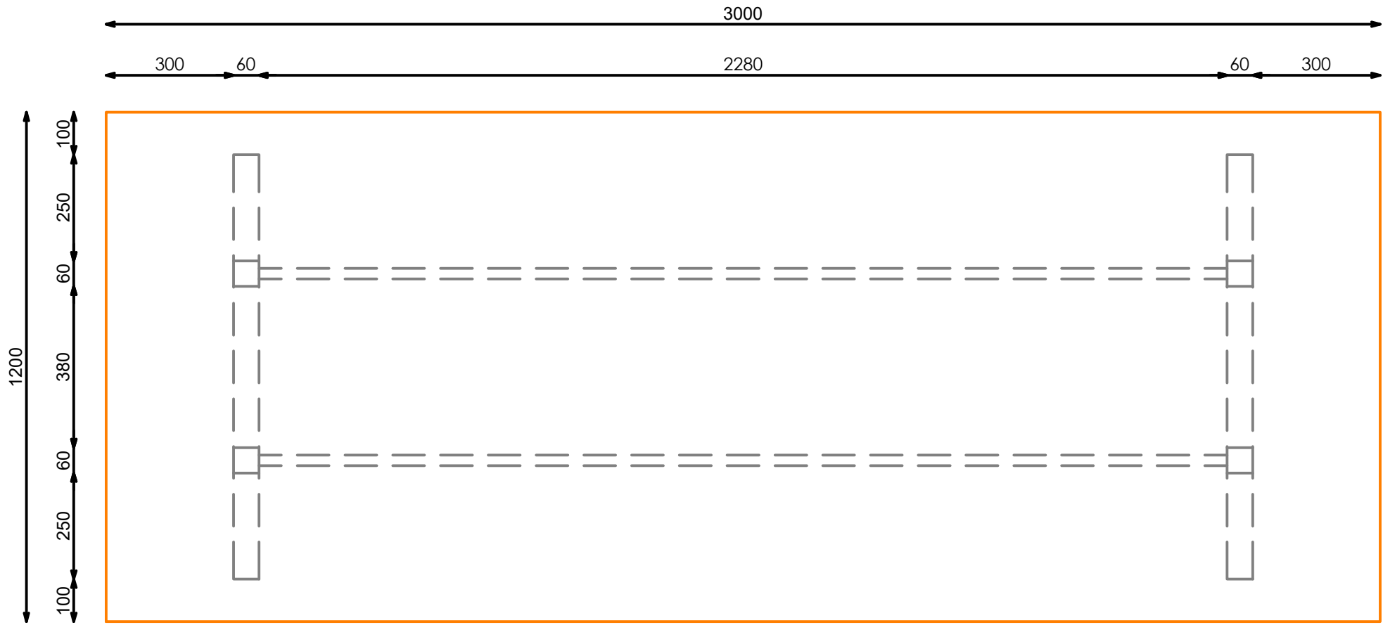
PLANTA SECCIONADA
