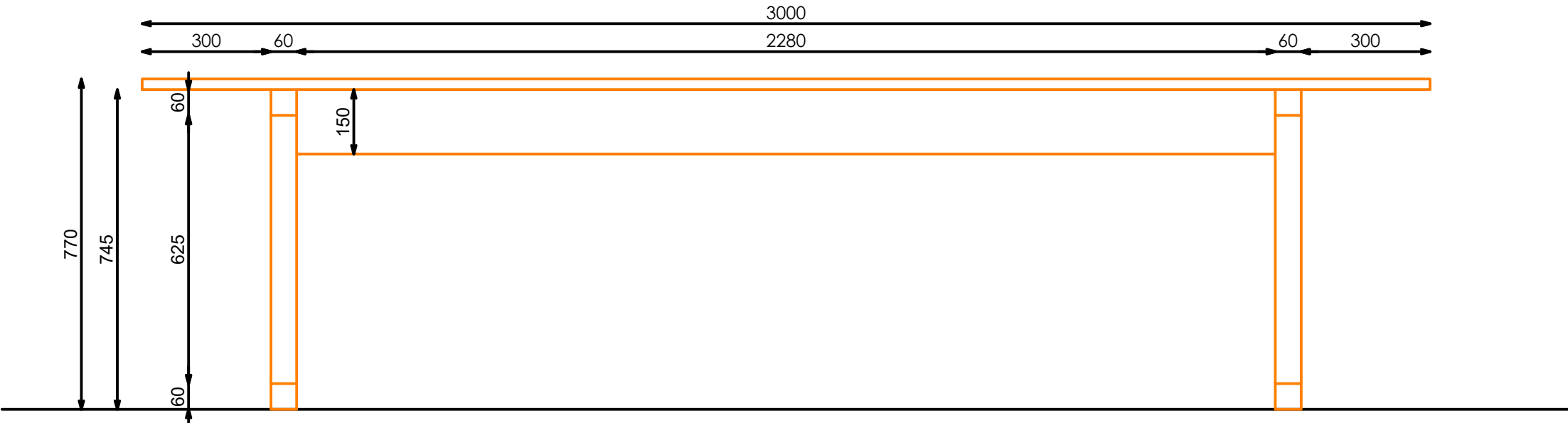
ALZADO FRONTAL
