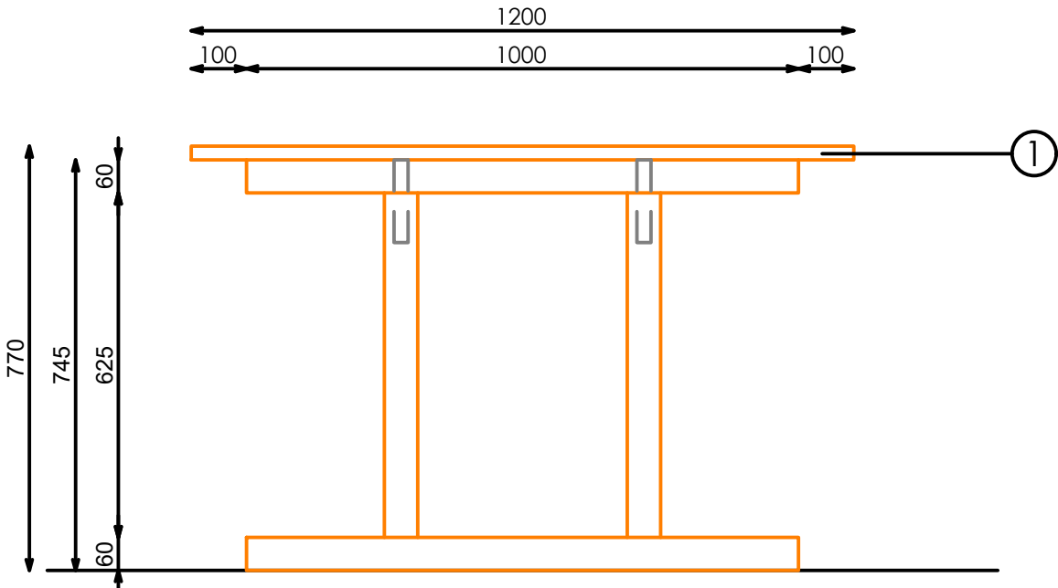
ALZADO LATERAL
