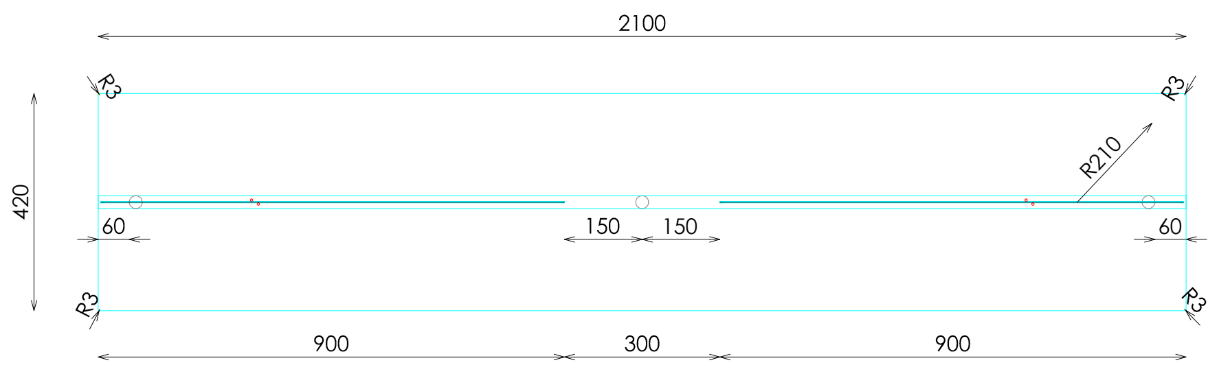
PLANTA
