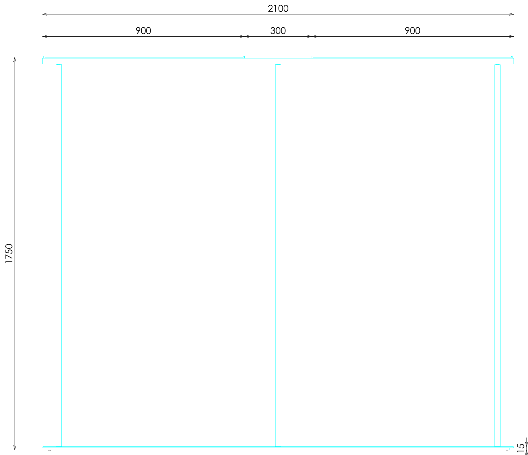
ALZADO
