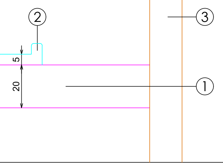
DETALLE C
