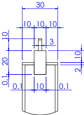
局部视图 AG 比例 1 : 2
