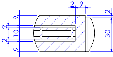
局部视图 AH 比例 1 : 2
