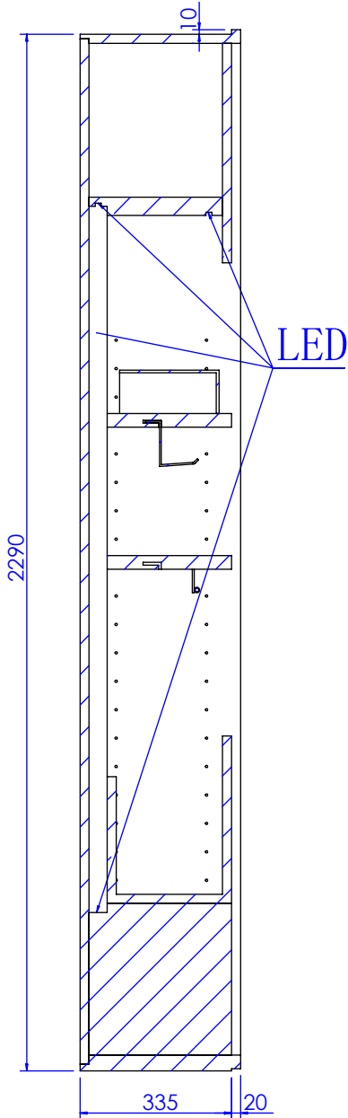
剖面 AG-AG
