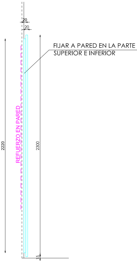
PERFIL
