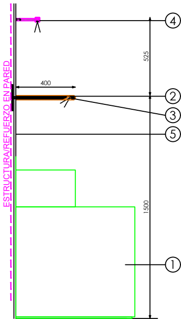
SECCIÓN BAKDAS
