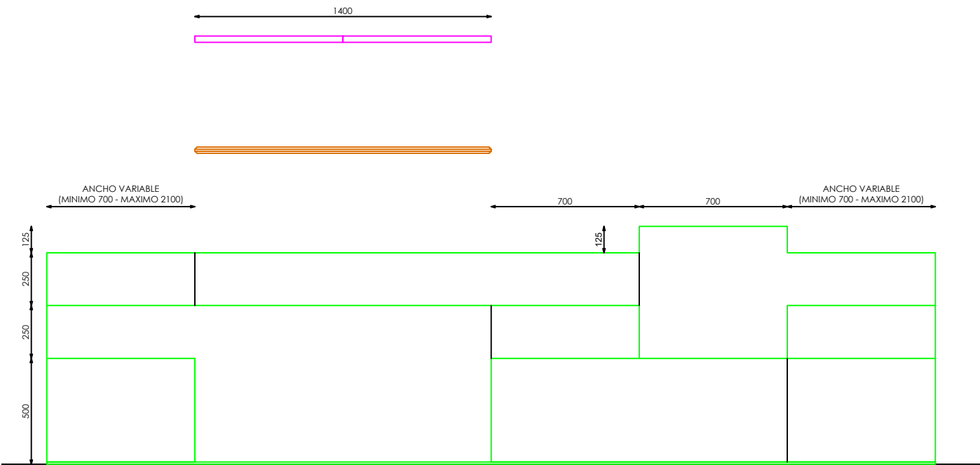
ALZADO FRONTAL
