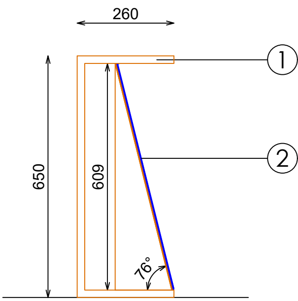
SECCIÓN
