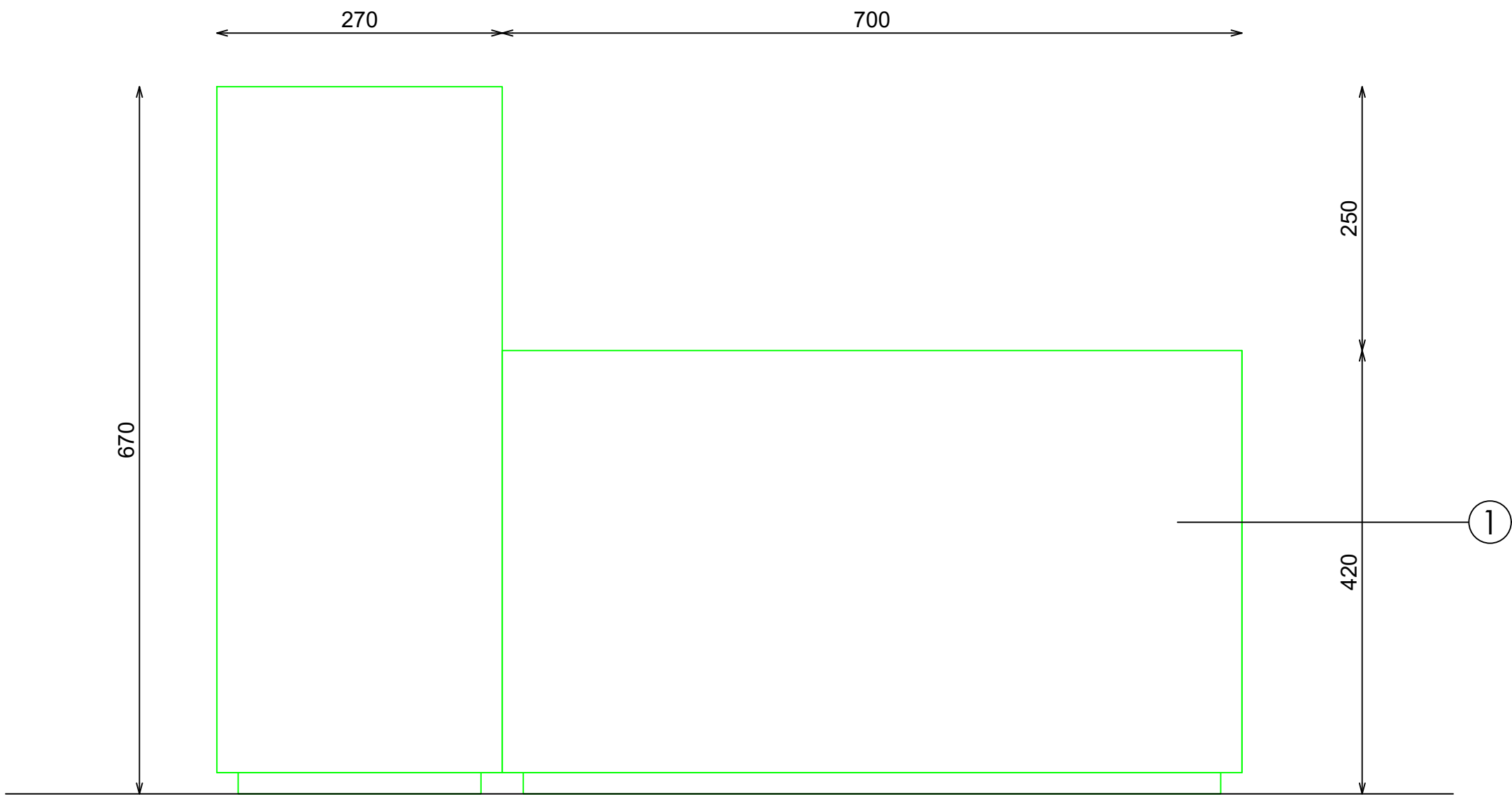
ALZADO
