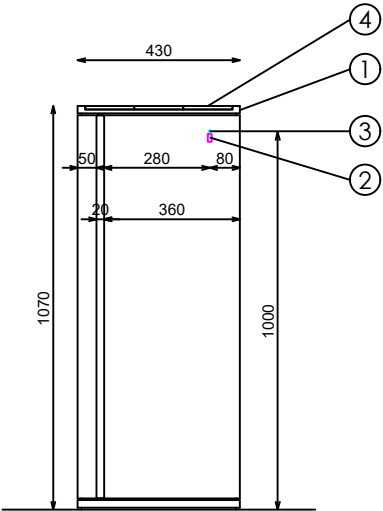
SECCIÓN
