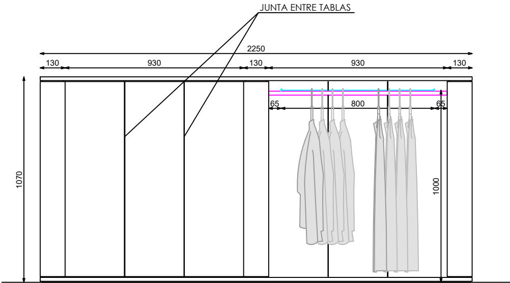
ALZADO
