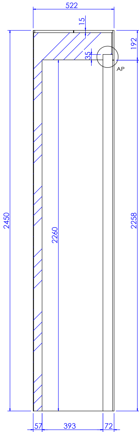
剖面 AK-AK
