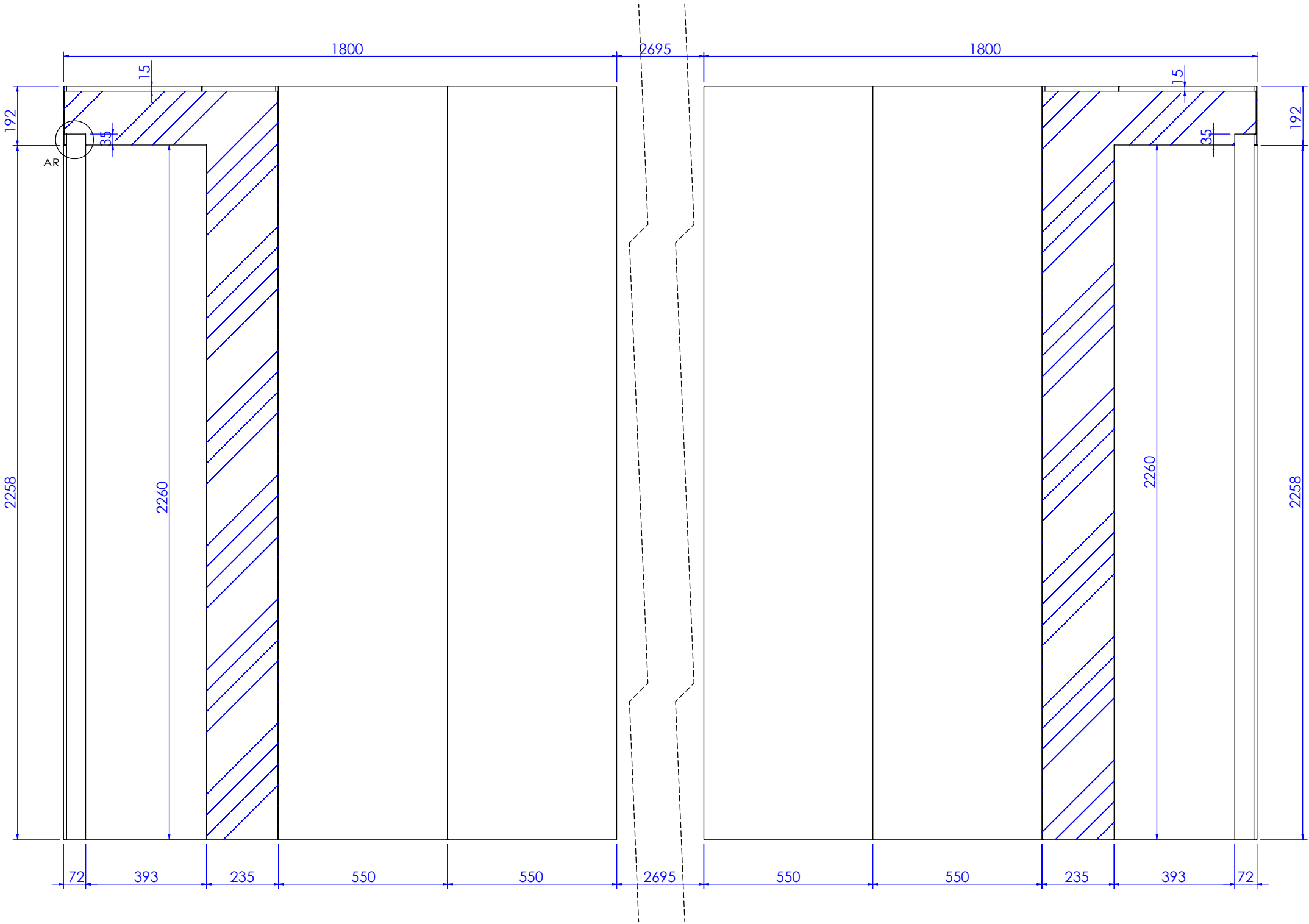
剖面 AM-AM
