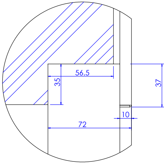
局部视图 AP 比例 1 : 2
