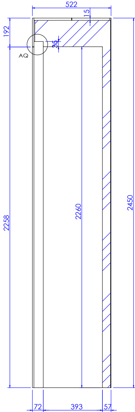
剖面 AJ-AJ
