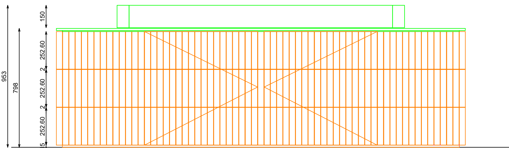
ALZADO POSTERIOR
