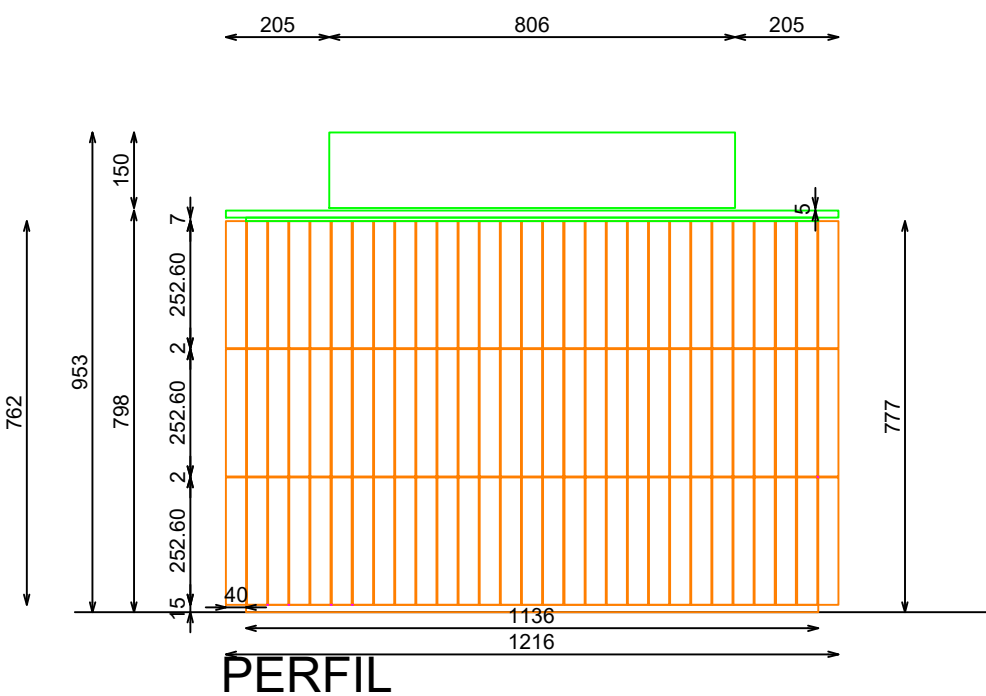
PERFIL
