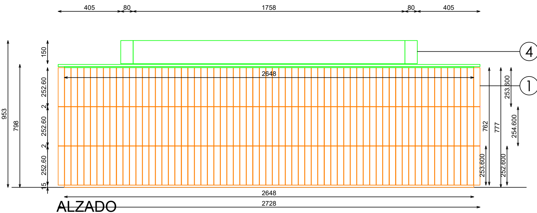
ALZADO
