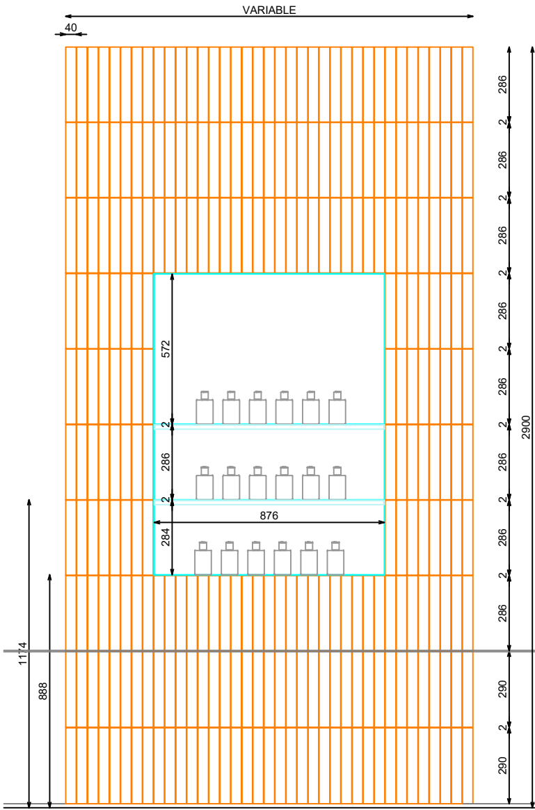
ALZADO FRONTAL
