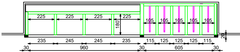
PLANTA A-A
