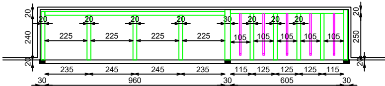
PLANTA B-B
