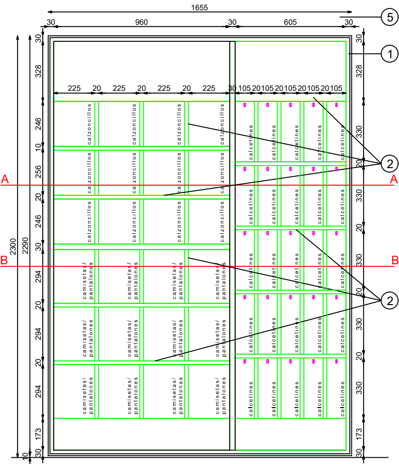
ALZADO FRONTAL
