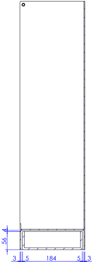
剖面 AG-AG
