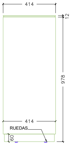
PERFIL SIDE ELEVATION
