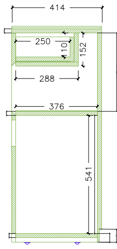
SECCIÓN BB' BB' SECTION
