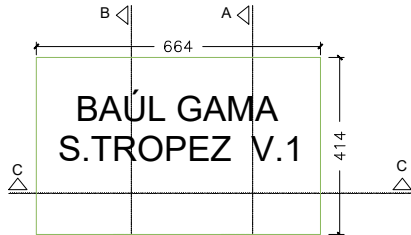
PLANTA PLAN
