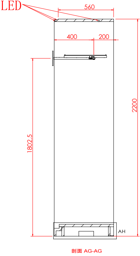
剖面 AG-AG
