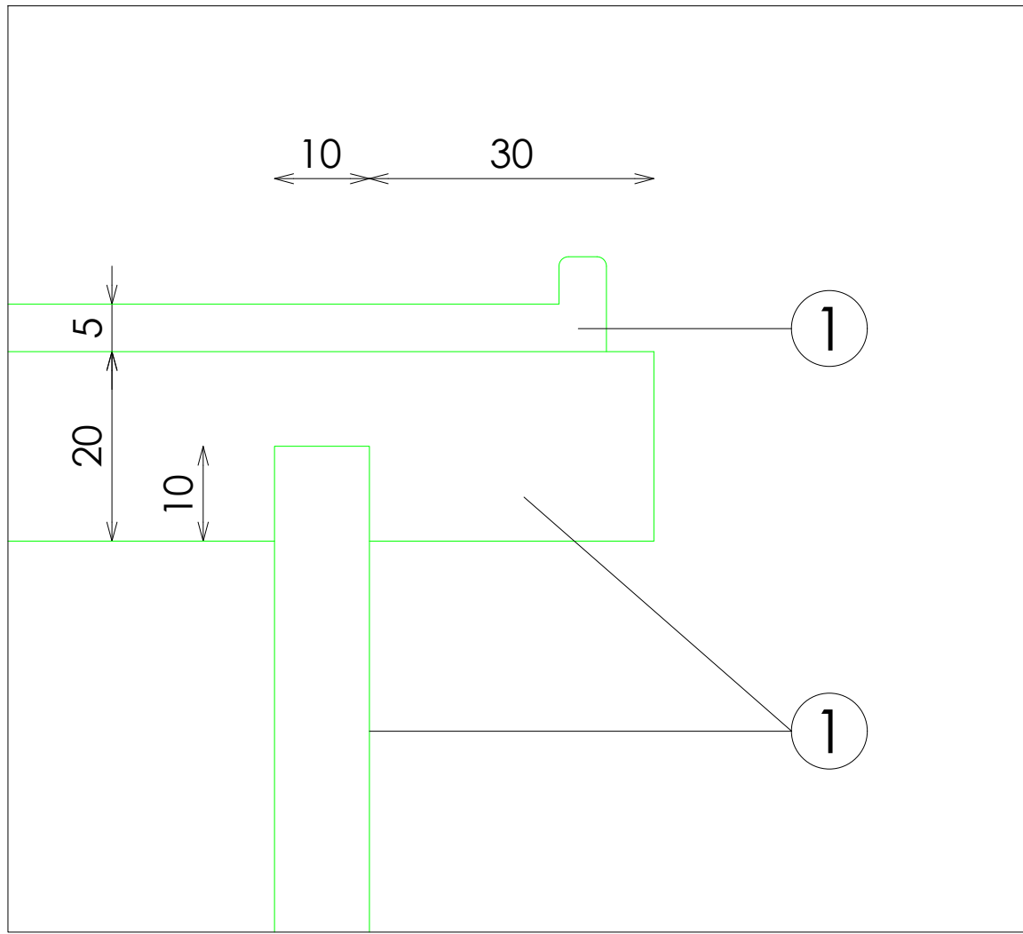
DETALLE C
