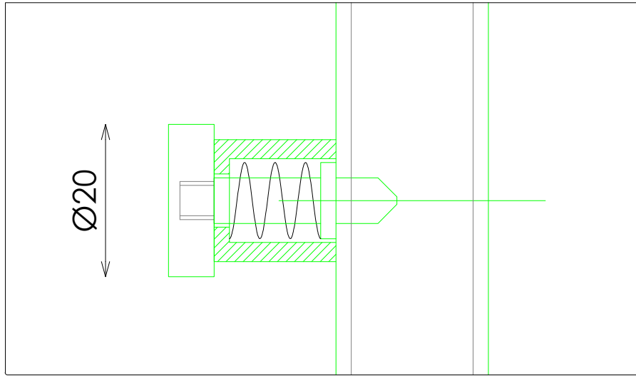
DETALLE SISTEMA ANCLAJE
