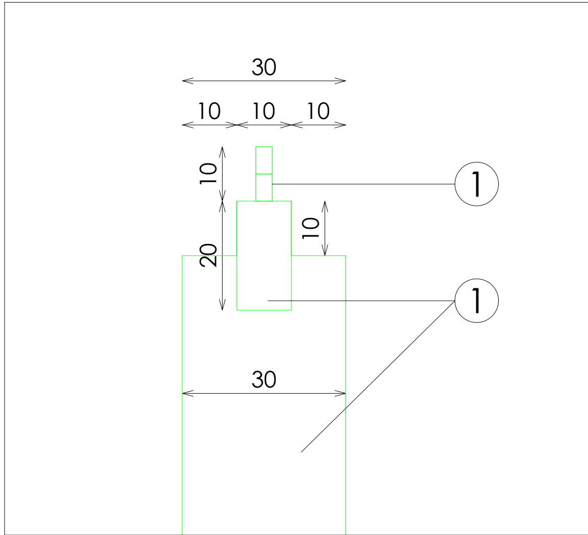
DETALLE A
