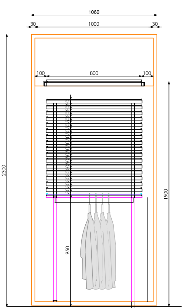
ALZADO
