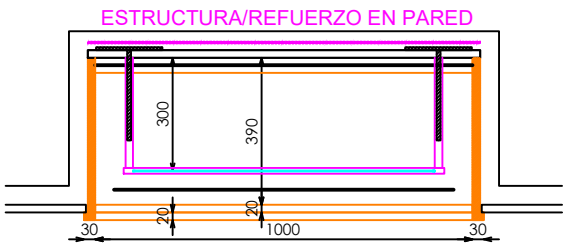
PLANTA BARRA
