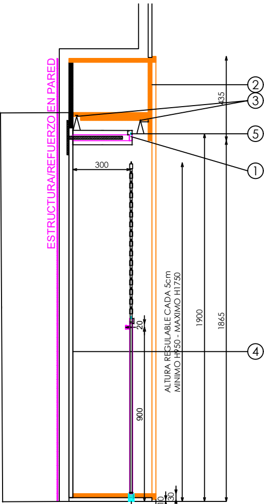
SECCIÓN
