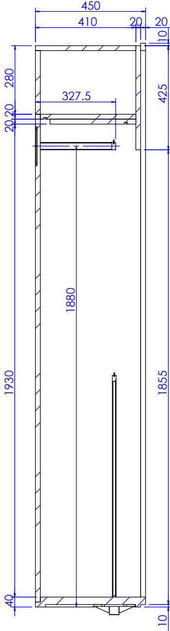
剖面 AI-AI
