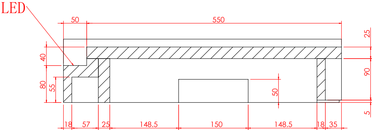
局部视图 AH 比例 1:5
