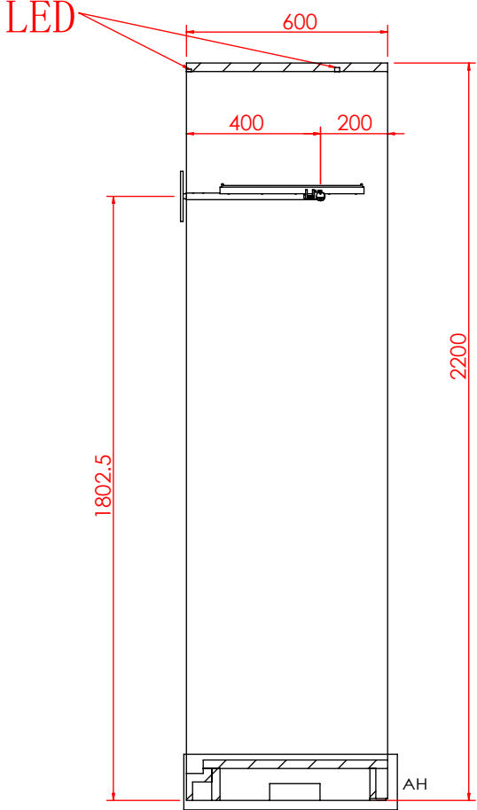
剖面 AG-AG
