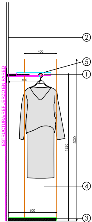
SECCIÓN
