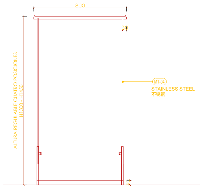
2 立面图 ELEVATION 1:10
