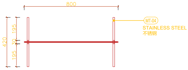
1 平面图 PLAN 1:10
