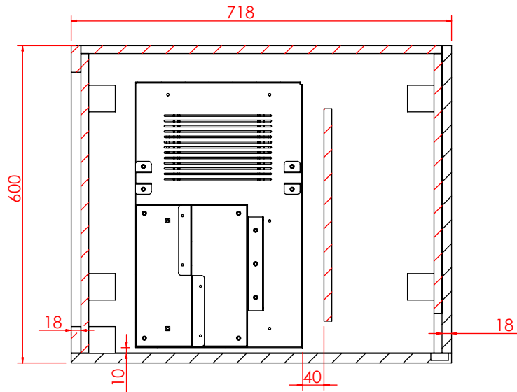
剖面 AG-AG
