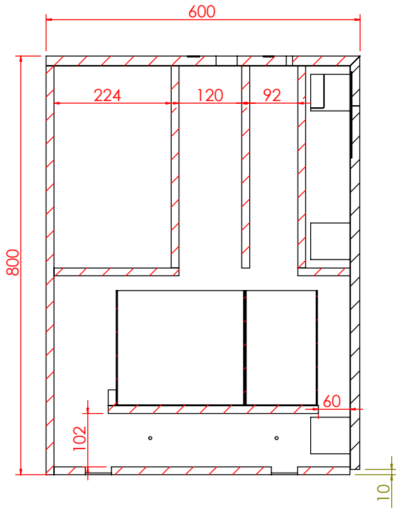
剖面 AI-AI
