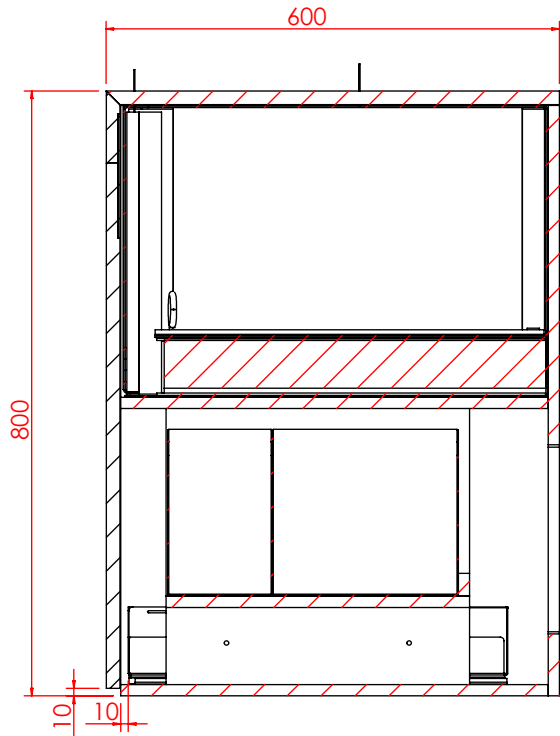
剖面 AH-AH
