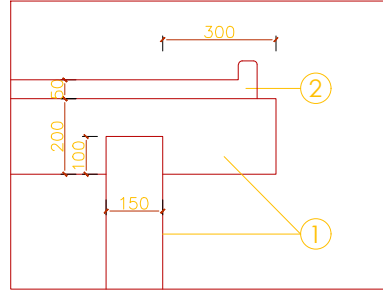
DETALLE C
