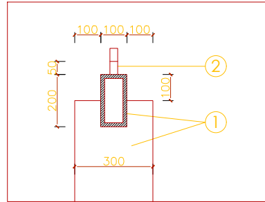
DETALLE B
