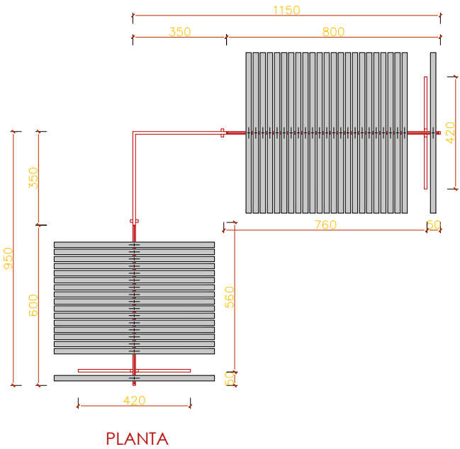
2 平面 1:10 PLAN
