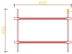
5 剖面图AA' 1:10 SECTION AA'
