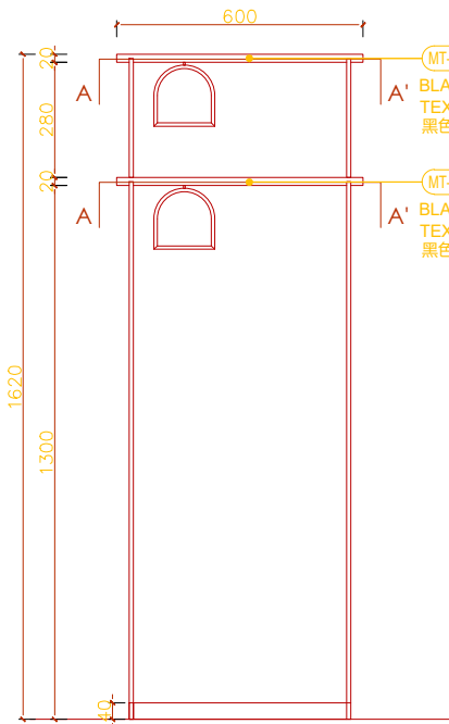
1 正立面 1:10 FRONT ELEVATION
