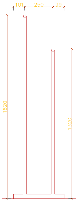
2 侧立面 1:10 SIDE ELEVATION
