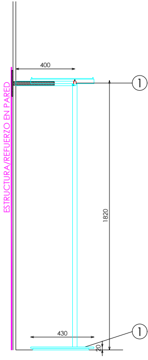
SECCION
