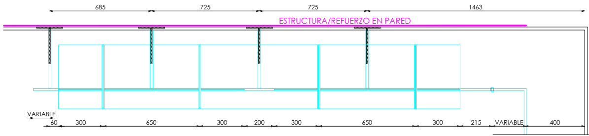
PLANTA
