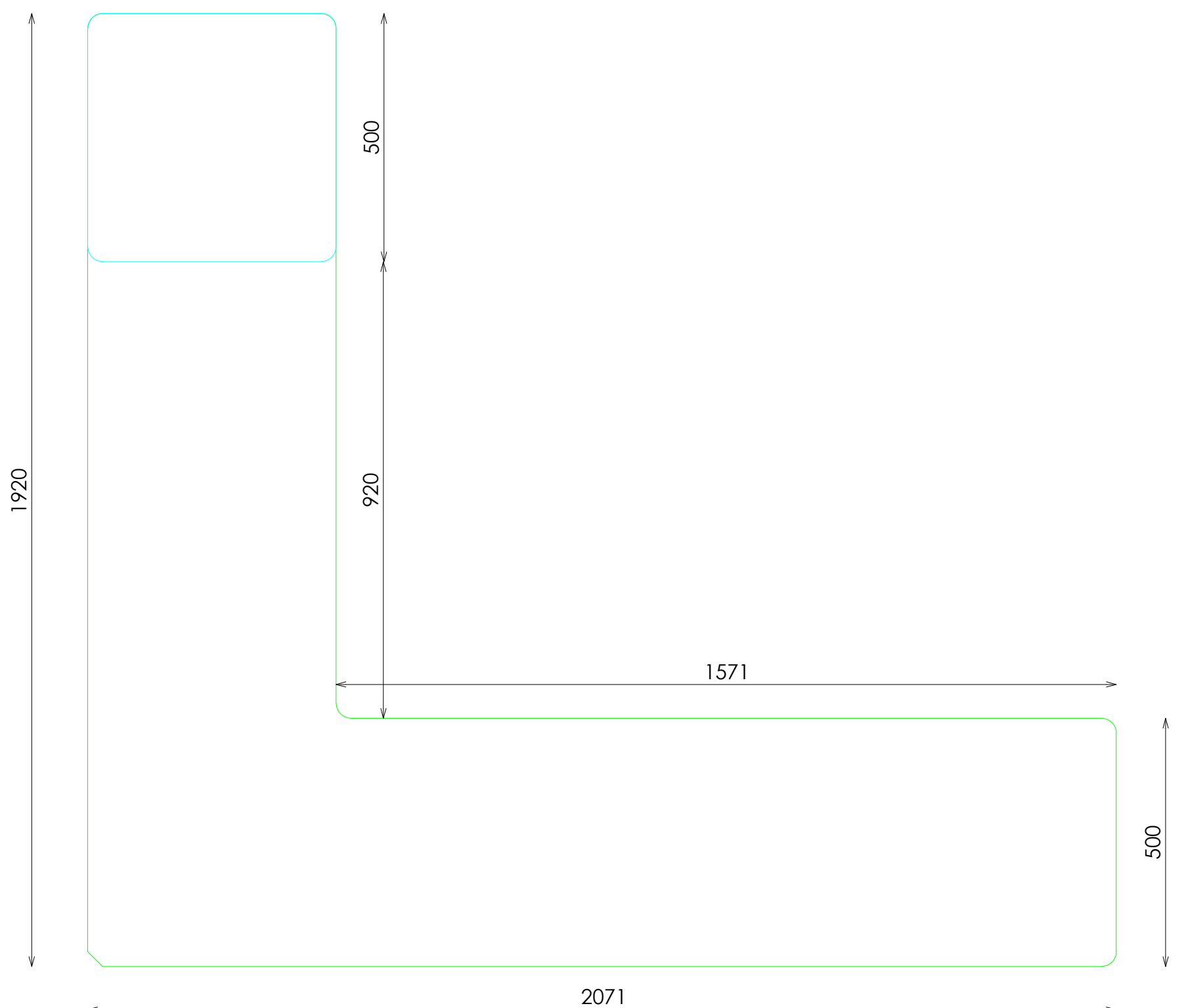
PLANTA
