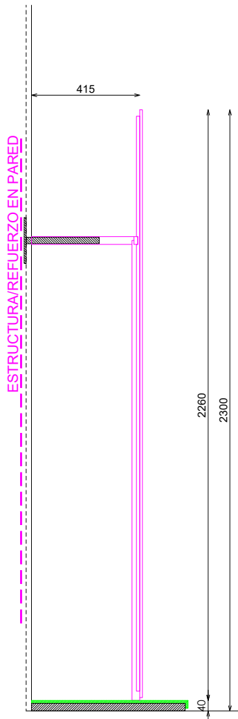
PERFIL
