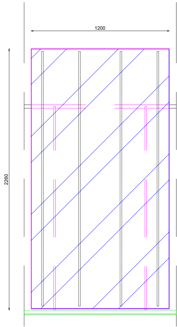
ALZADO CONJUNTO
