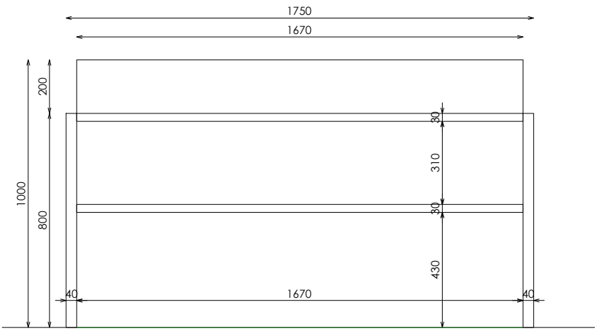
ALZADO FRONTAL
