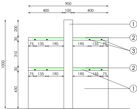
SECCION
