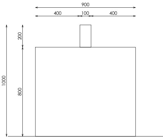
ALZADO LATERAL
