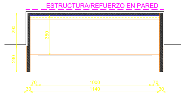
PLANTA
