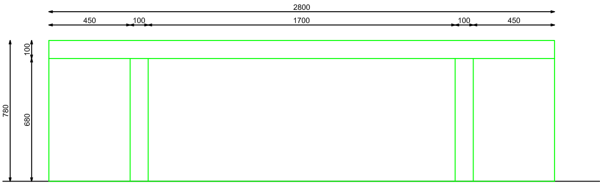
ALZADO FRONTAL
