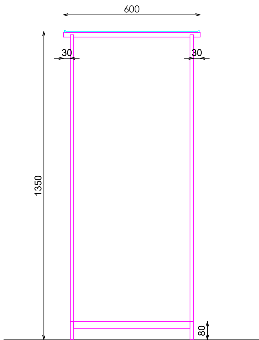
ALZADO
