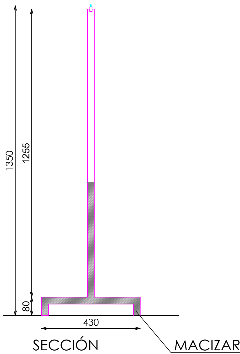
SECCIÓN
