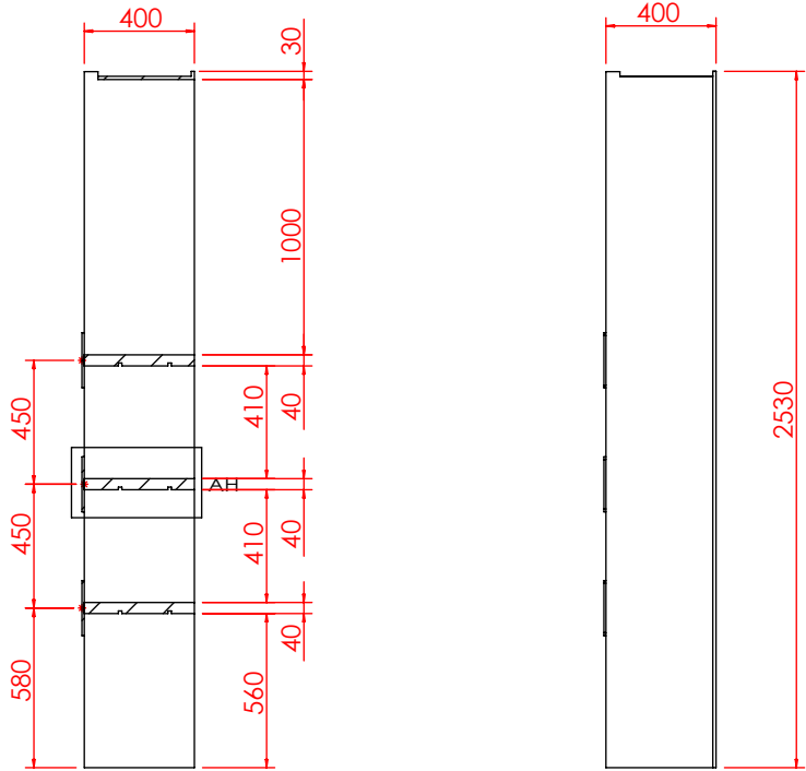
剖面 AG-AG
