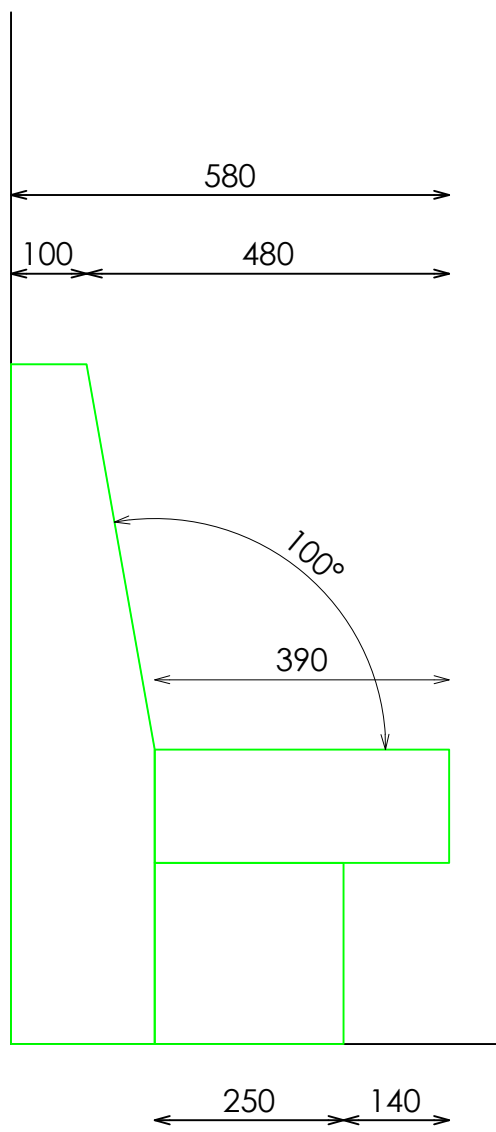
PERFIL
