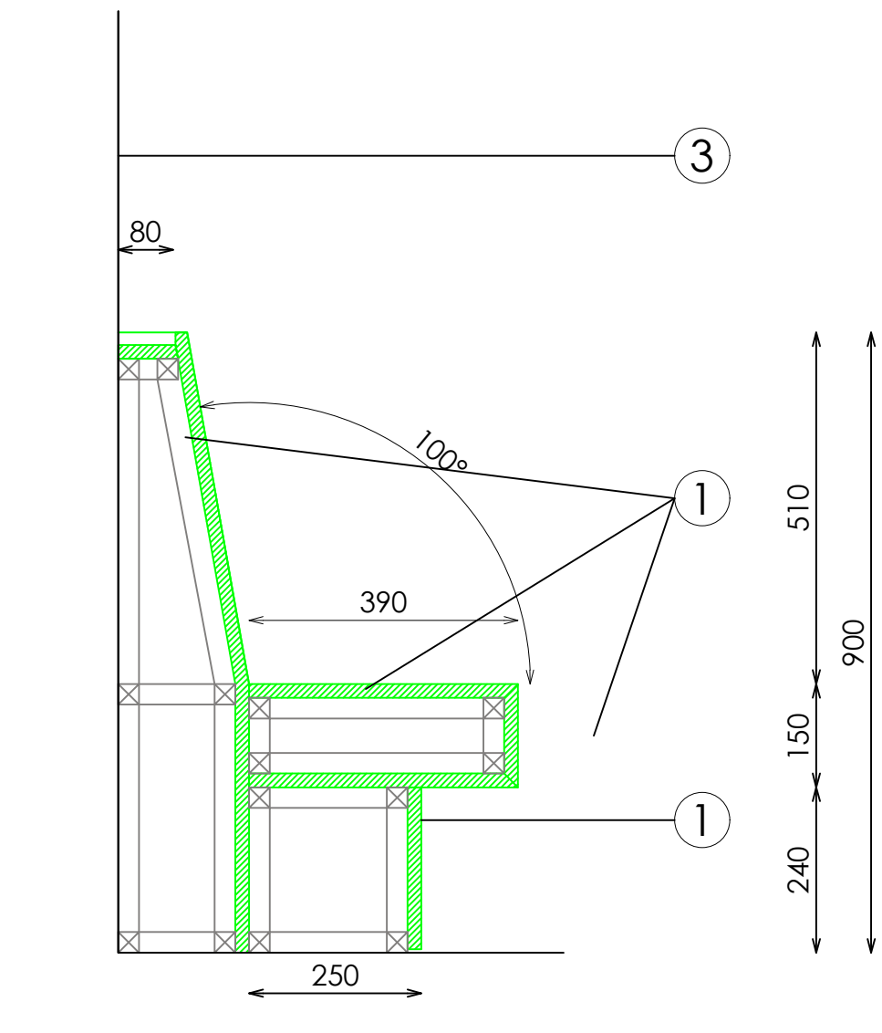
SECCION
