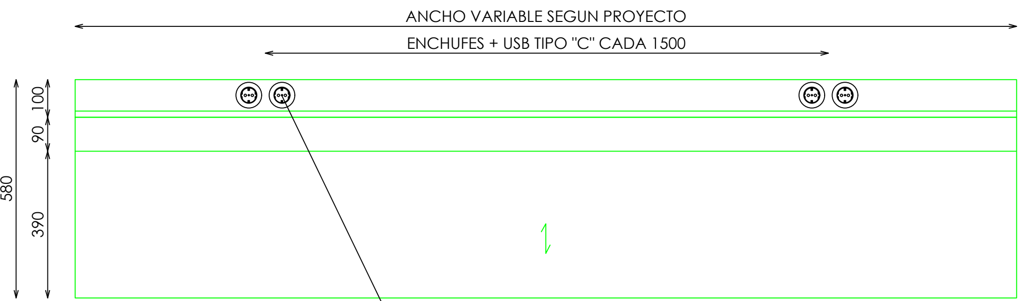
PLANTA
