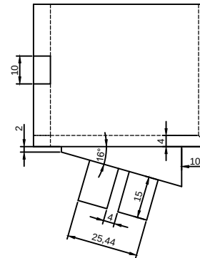
PERFIL
