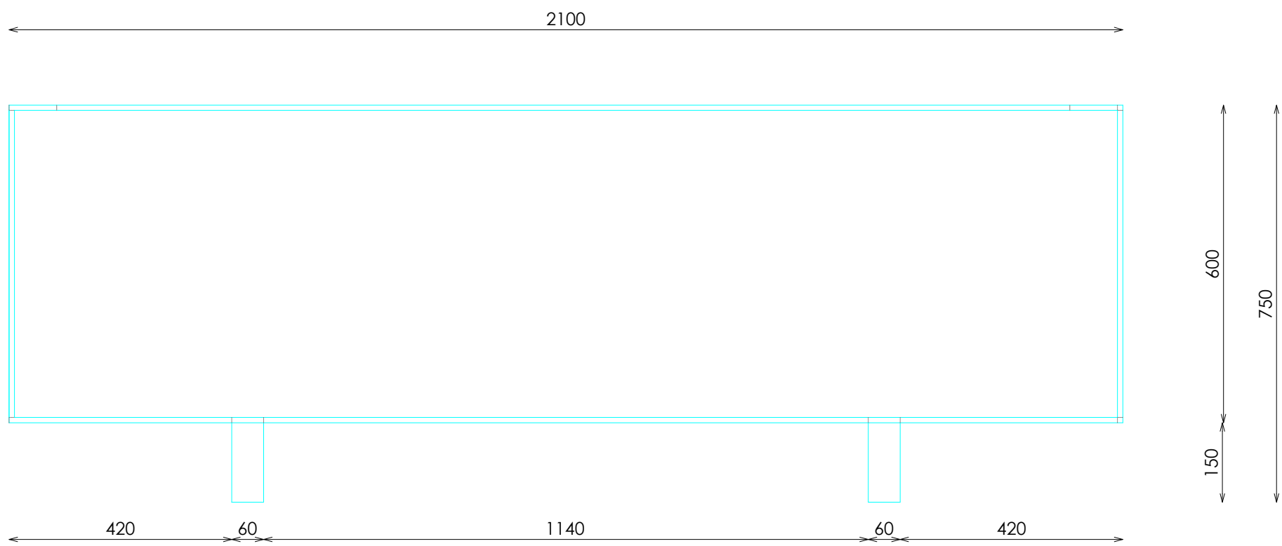
ALZADO FRONTAL
