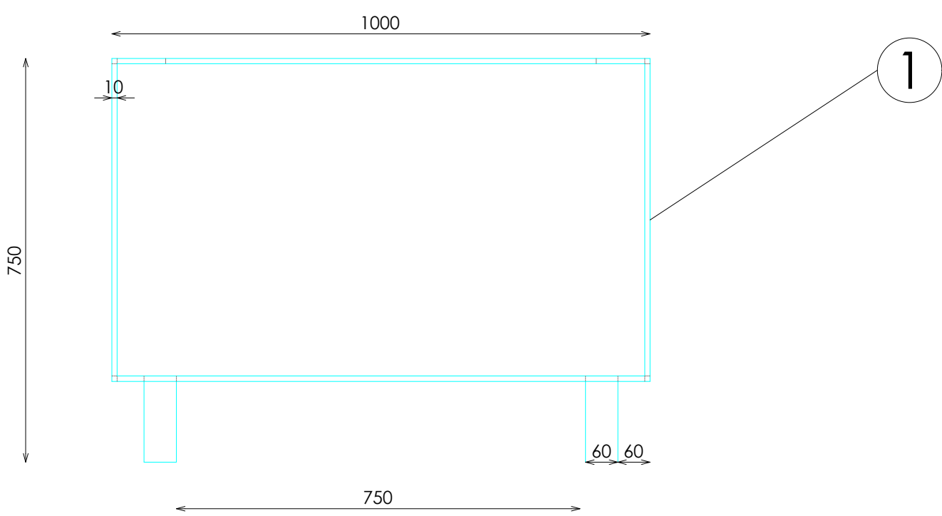
ALZADO LATERAL
