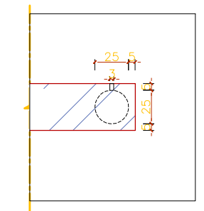
4 1:2 节点 DETAIL
