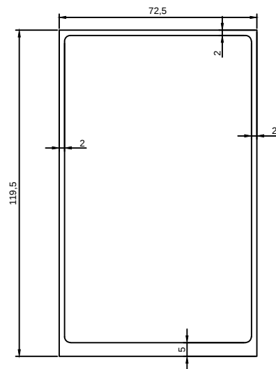
PLANTA
