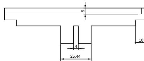
SECCIÓN PERFIL
