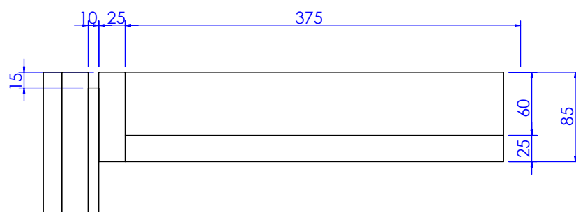
局部视图 AG 比例 1 : 5
