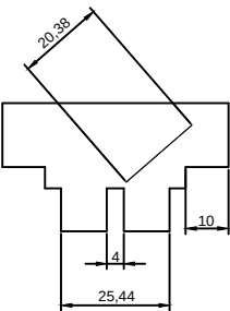
SECCIÓN PERFIL
