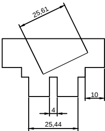
SECCIÓN PERFIL
