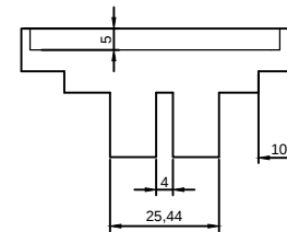
SECCIÓN PERFIL
