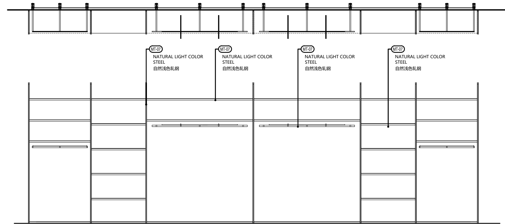
1 平面 SECTION 1:20
